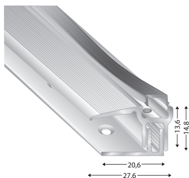
inkl. Grundprofil / Base profile 7100
