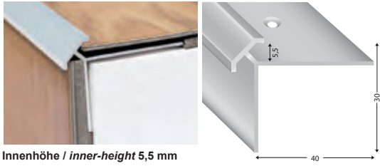
Innenhöhe / inner-height 5,5 mm
