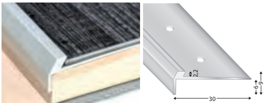
Innenhöhe / inner-height 2,2 mm
